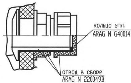
A-A (установка отвода) M1:1
