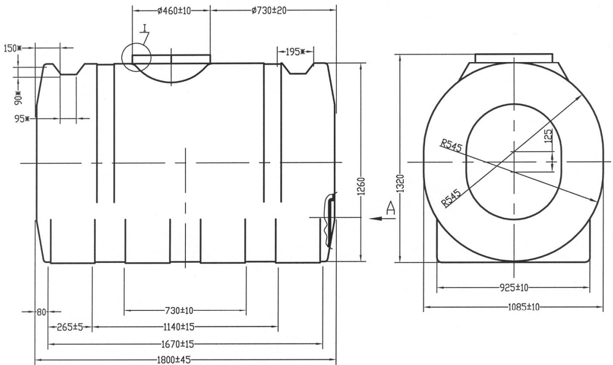
Вид А
