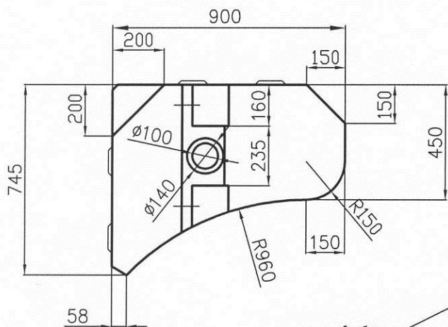
промыв. бак V=300 л.
